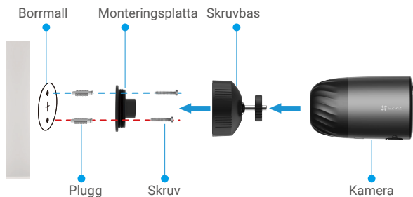
Fig. 1 Säker med skruvbaser
