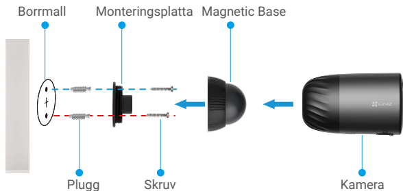
Fig. 2 Säker med magnetisk bas
